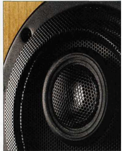
Nicht ganz (ko-)axial: Der Hochtöner ist etwas außermittig im Gitter des Tiefmitteltöners verbaut und hat einige Zentimeter Sicherheitsabstand zum Konus.
