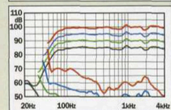
Neutral und tief reichend, minimal wellig, erkennbare Bündelung. Geringer Klirr, nur leichte Spitze um 2 kHz.
